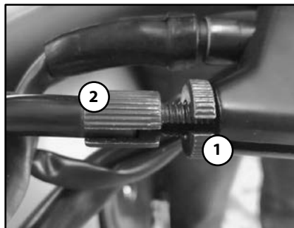
1. Abrazadera del embrague 2. Tornillo embrague
