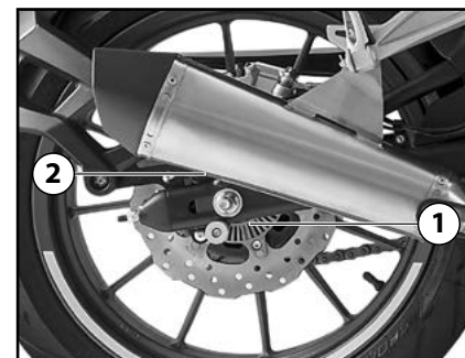
1. Rotor de capteur arrière 2. Capteur de roue arrière
